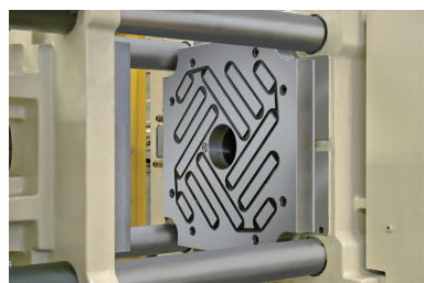
M-TECS 120 mágneses rögzítőrendszerek műanyag fröccsöntő gépekhez 120 °C-ig
