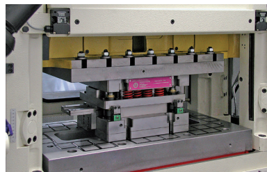
M-TECS 80 mágneses rögzítőrendszerek lemezalakításhoz 80 °C-ig
