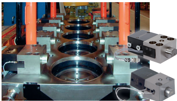
5-állomású kovácsgép felszerelve ékes szorítóelemekkel (ülékes-szelepekkel) az egyes állomások külön vezérléséhez
