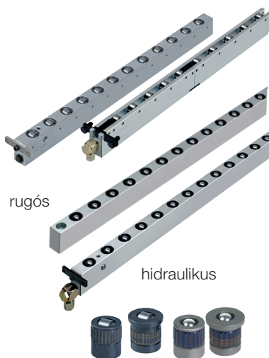
Görgős- és golyóslécek vagy betétek
